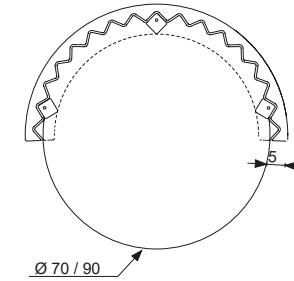
Ecran de séparation Ø70/90 x H.65 cm
