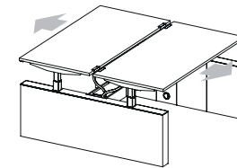
Bench électrique à plateaux coulissants, pied panneau avec passe câbles horizontal et vertical
