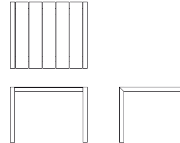
Fixe à lattes prof. 136 cm. L. 139 cm - Dispo. en Fenix-NTM®
