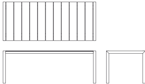
Fixe à lattes prof. 90 cm. L. 161 / 180 / 215 / 270 cm - Dispo. en Fenix-NTM®
