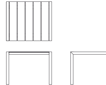
Fixe à lattes prof. 136 cm. L. 139 cm - Dispo. en Fenix-NTM®
