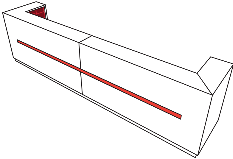
Banque vue de face L.290 / 330 / 370 / 410 x P.108,5 x H.100 cm
