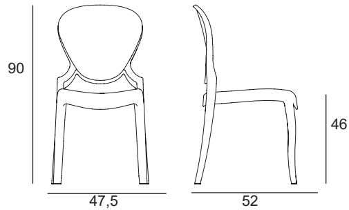
Chaise Queen 650 en polycarbonate opaque ou transparent
