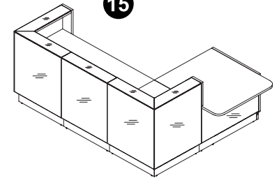
Droit ou gauche L.255/275 x P.185 cm
