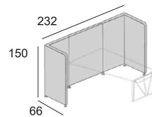
Alcôve pour table asymétrique P.100 x H.74 cm
