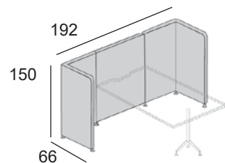
Alcôve pour table rectangle P.60 x H.100 cm
