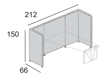
Alcôve pour table asymétrique P.80 x H.74 cm
