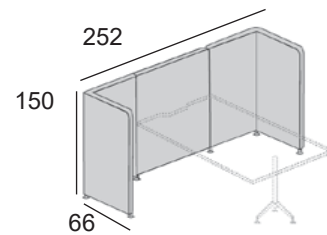
Alcôve pour table asymétrique P.120 x H.74 cm
