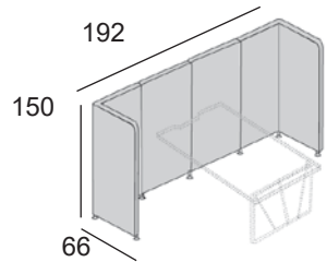
Alcôve pour tables rectanglées P.60/80/100/120 x H.74 cm
