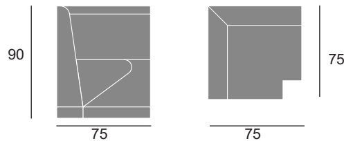
Module d'angle L.75 x P.75 x H. 90 cm
