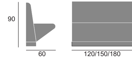
Module L.120 ou 150 ou 180 x P.60 x H. 90 cm
