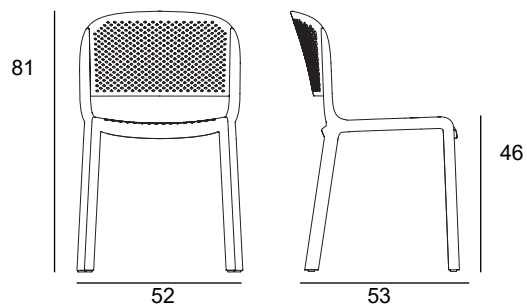
DOMÉ 261 L.52 x P.53 x H.81 cm, hauteur d'assise 46 cm
