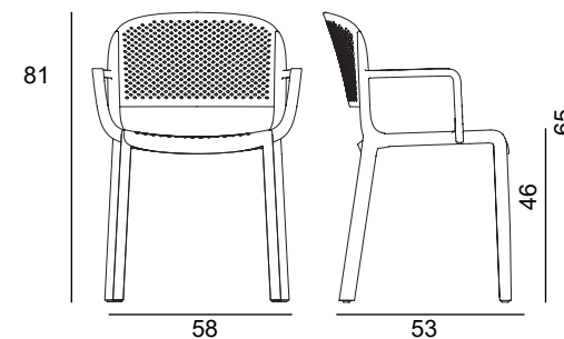
DOMÉ 266 L.58 x P.53 x H.81 cm, hauteur d'assise 46 cm
