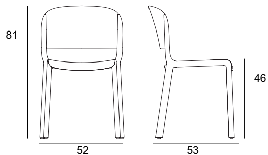
DOME 260 L.52 x P.53 x H.81 cm, hauteur d'assise 46 cm
