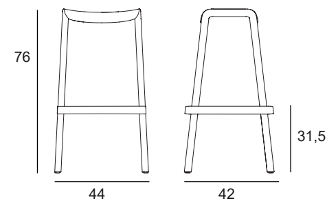
DOMÉ 268 L.44 x P.42 x H.76 cm
