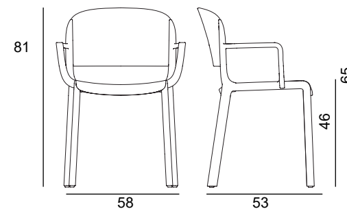
DOME 265 L.58 x P.53 x H.81 cm, hauteur d'assise 46 cm
