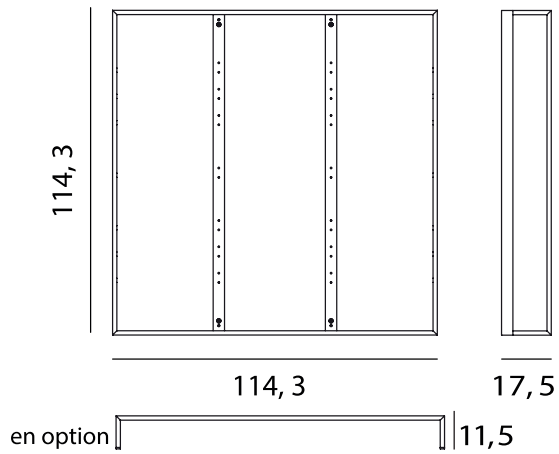
Module 1 L.114,3 x P.17,5 x H.114,3 cm
