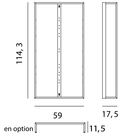
Module 2 L.59 x P.17,5 x H.114,3 cm
