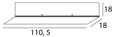
A 01 L.110,5 x P.18 x H.18 cm
