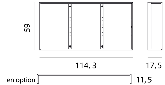
Module 3 L.114,3 x P.17,5 x H.59 cm
