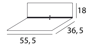
B 03 L.110,5 x P.36,5 x H.18 cm
