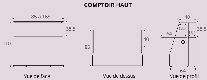
COMPTOIR HAUT ANGLE 90°
