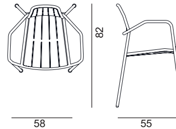
Chaise Osmo Alu L.58 x P.55 x H.82 cm
