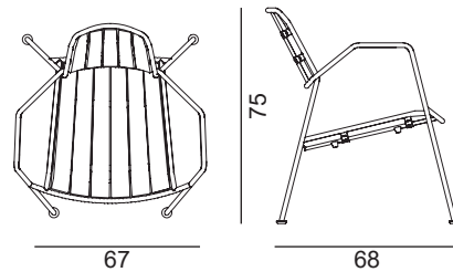
Fauteuil Osmo L.67 x P.68 x H.75 cm
