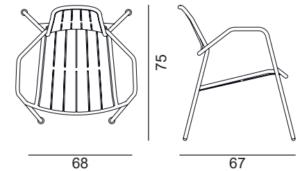
Fauteuil Osmo Alu L.68 x P.67 x H.75 cm
