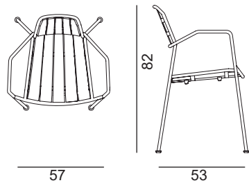
Chaise Osmo L.57 x P.53 x H.82 cm
